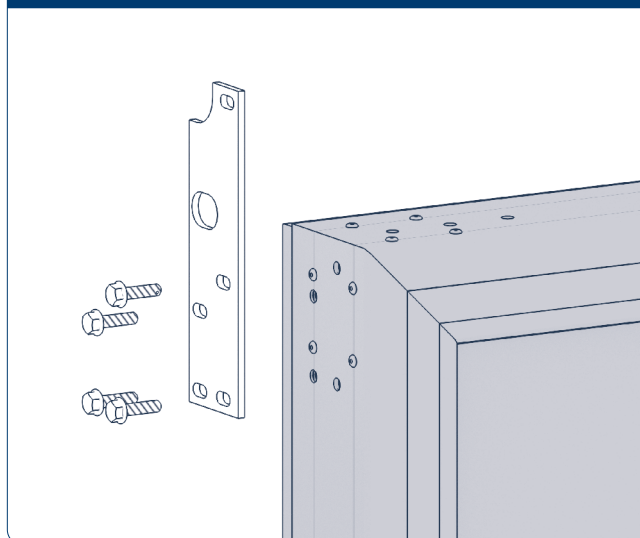
Рис. 3. Вид В
